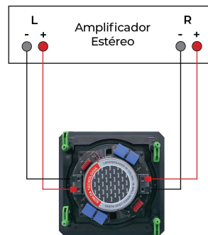
LIGAÇÃO DE 1 FALANTE POR ZONA
