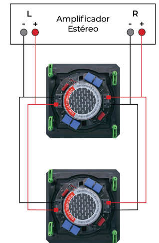
LIGAÇÃO DE 2 FALANTES POR ZONA
